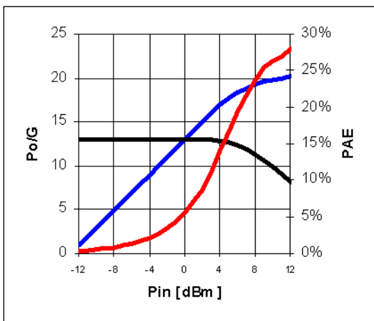
900MHz, 5V/70mA
